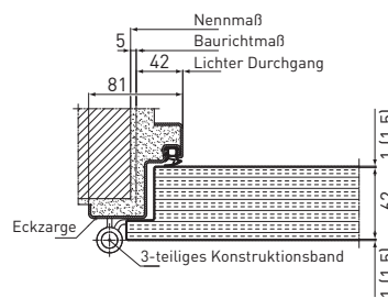
Horizontalschnitt 1-flgl.
